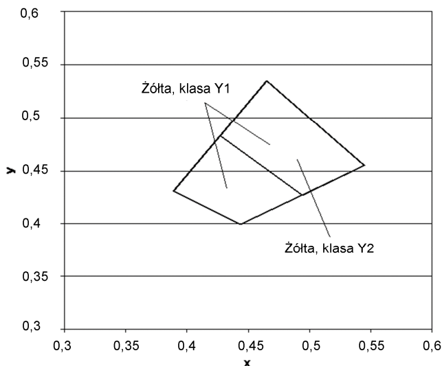
Rys.2. Współrzędne chromatycyjnosc x,y dla barwy żółtej oznakowania
